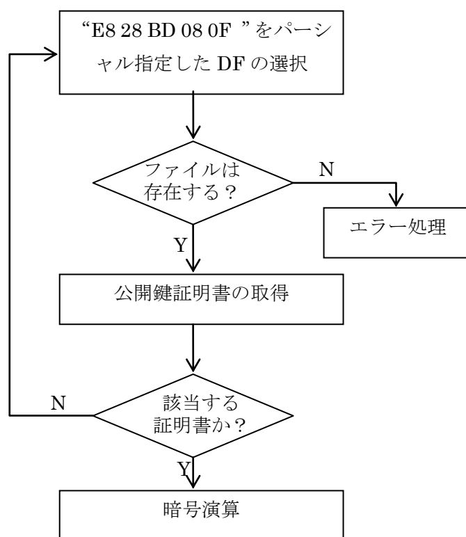
図 A.1 JIS X 6320-15 に従った PKI カードアプリケーションの検索と利用
