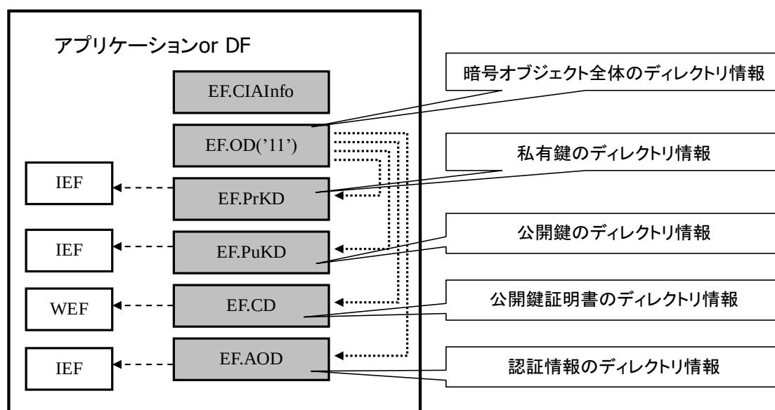
図4 JIS X 6320-15 の基本構成
