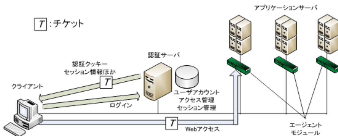
図4. エージェント方式
