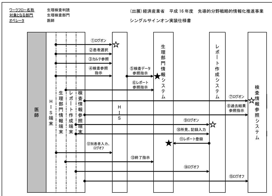
図14. 生理検査判読ワークフロー
