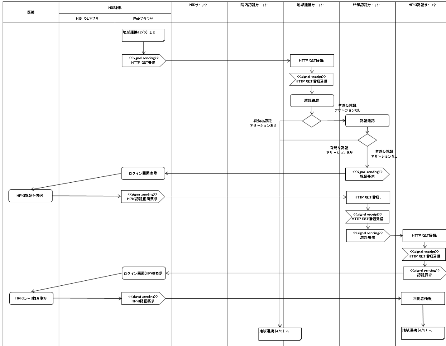
付図6. 病病連携時の他院診療情報参照：アクティビティ図（SSO 導入後） 3/5
