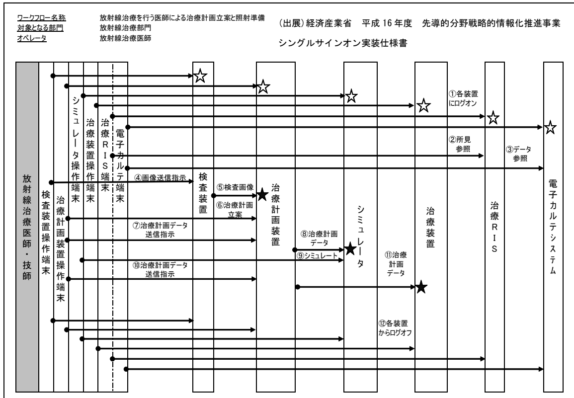
図 1 3. 放射線治療を行う医師による治療計画立案と照射準備ワークフロー
