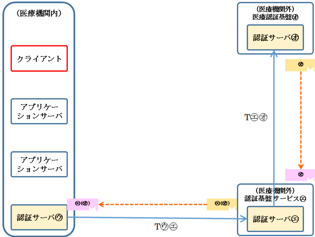
図 1 8. 医療機関外サイトとの信頼関係の組合せイメージ (Case1)
