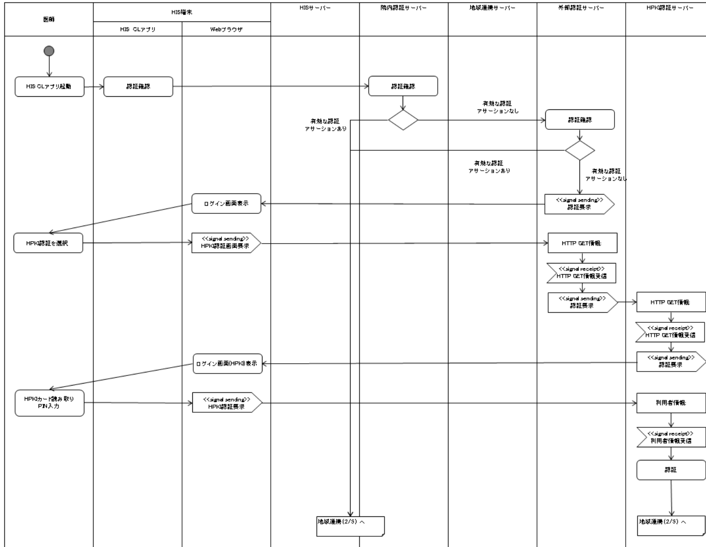
図 28-1. 病病連携時の他院診療情報参照：アクティビティ図 1/5
