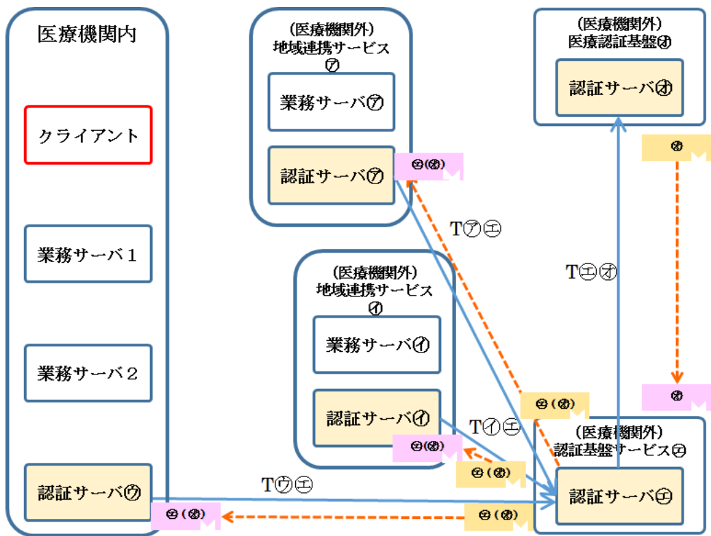
図 2 1. 医療機関外サイトとの信頼関係の組合せイメージ (Case3-1)
