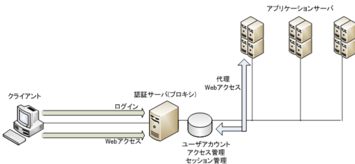
図3. リバースプロキシ方式
