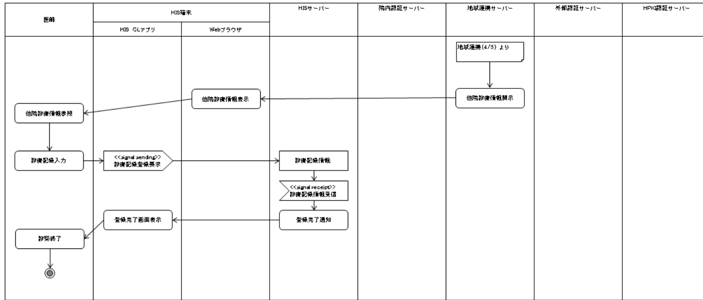
図 2 8 - 5 . 病病連携時の他院診療情報参照 : アクティビティ図 5/5
