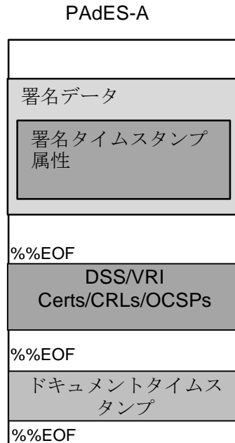
図 6.5.3 PAdES-A プロファイルの PDF データ構造のイメージ
