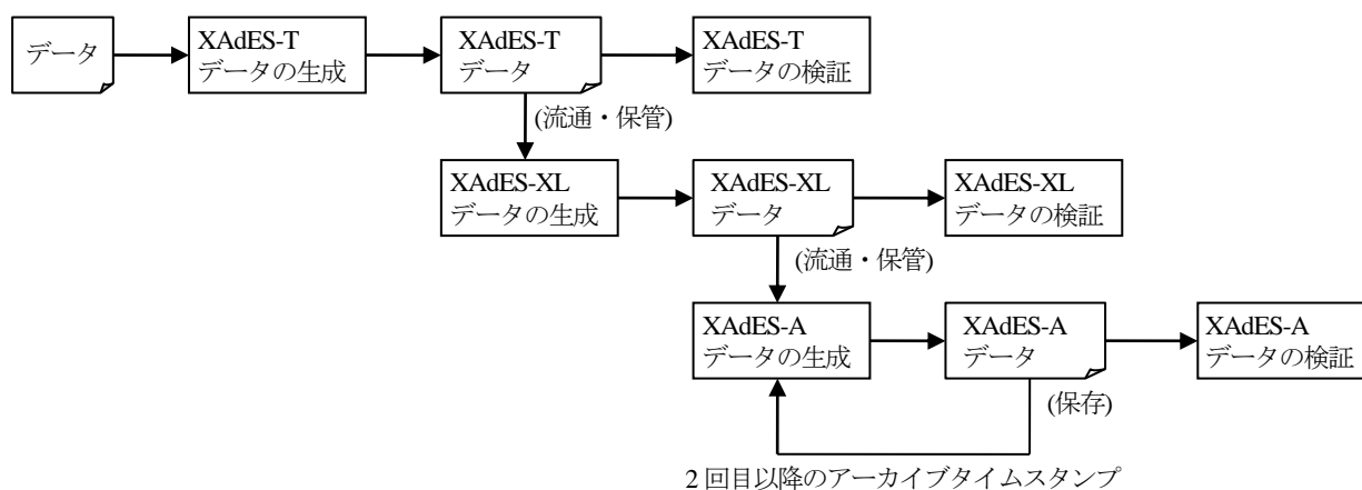
図 6.4.1 XAdES-Tデータ、XAdES-XLデータ、及びXAdES-Aデータとの関係
