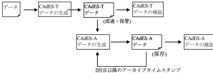
図 6.3.1 CAdES-TデータとCAdES-Aデータとの関係
