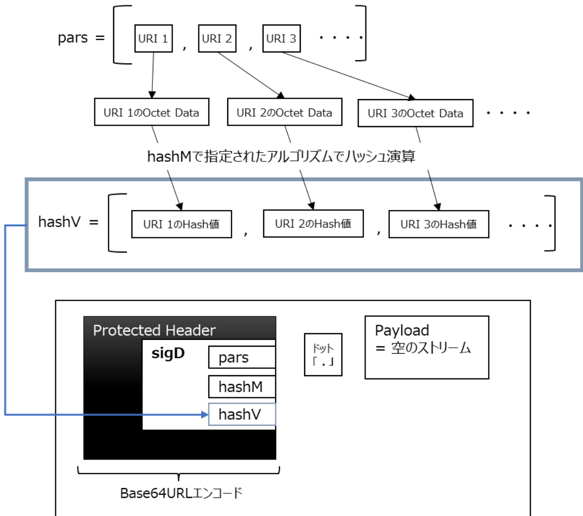
図 6.6.6 ObjectIDByURIHash の場合の構造
