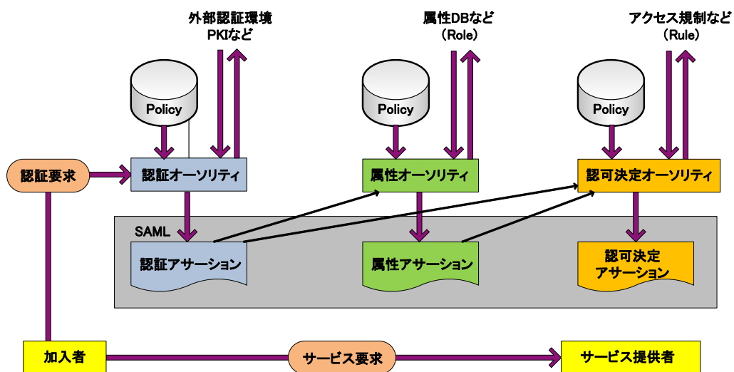
図6. SAML 方式
